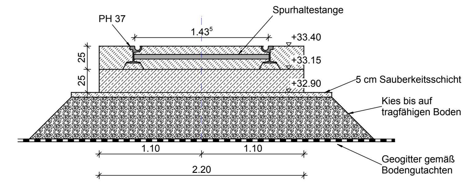
Querschnitt 1:25
